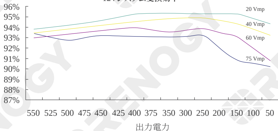
12Vシステム変換効率
