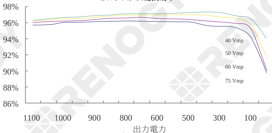
24Vシステム変換効率
